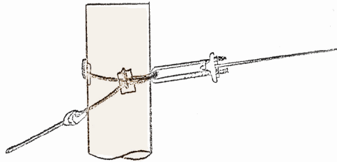
Stagets infästning i stagstolpe för portstag (överstagning)
